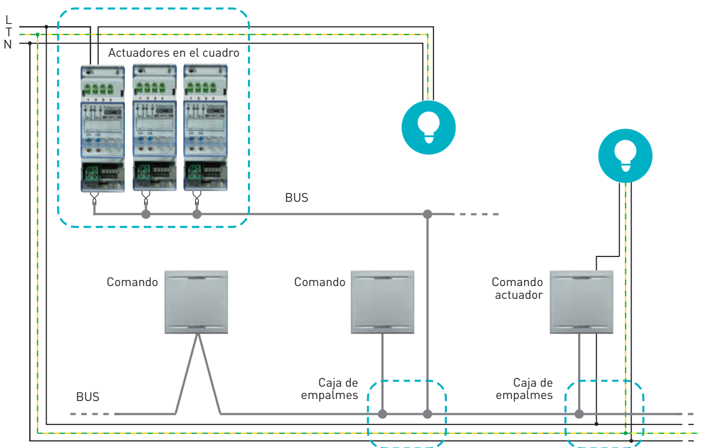
Ejemplo de cableado del sistema de iluminación
